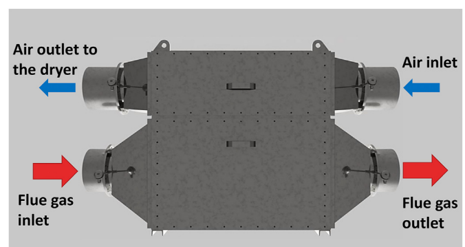
Fig. 4. HPHE system.
