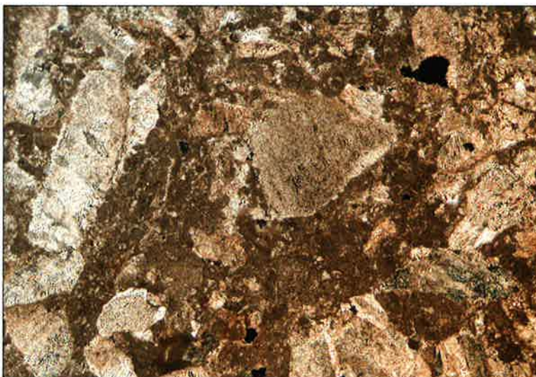
tav. 16b. Pietra di Aurisina, varietà granitello al microscopio ottico, base di stele esposta nel parco Novi Ark. Luce trasmessa, nicol incrociati, lato lungo dell'immagine = 5,33 mm.
