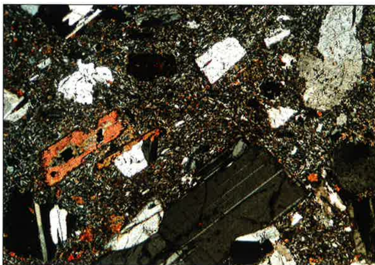
tav. 16c. Trachite euganea al microscopio ottico, stele di Stazio Gavidio Secondo esposta nel parco Novi Ark. Luce trasmessa, nicol incrociati, lato lungo dell'immagine = 5,33 mm.
