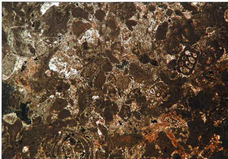
tav. 16a. Pietra di Vicenza al microscopio ottico, numero di reperto 42, US 81. Luce trasmessa, nicol incrociati, lato lungo dell'immagine = 5,33 mm.
