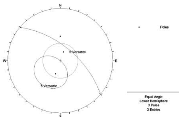
Fig. 7.6 - Test di Goodman per lo scivolamento (scarpata laterale della cava "Il Pescale")
