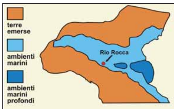
Fig. 5.4 – Ricostruzione dell'Italia centro-settentrionale durante il Pliocene (modificata da Vai, 1988)
