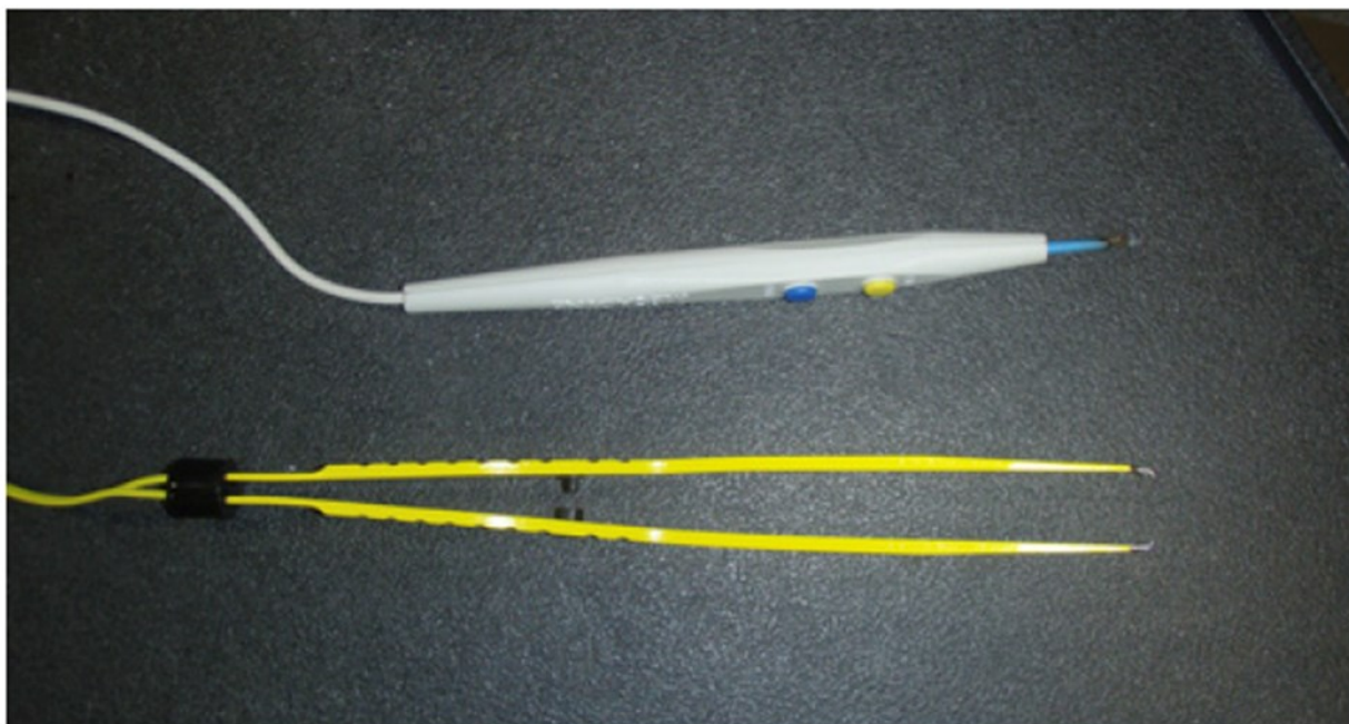
Figura 4 Unità elettrochirurgica: elettrodi attivi e di ritorno, e cavi di collegamento (Da: Guida non vincolante di buone prassi per l'attuazione della Direttiva 2013/35/UE relativa ai campi elettromagnetici. Volume 2: Studi di casi. Commissione europea. Direzione generale per l'Occupazione, gli affari sociali e l'inclusione. Unità B.3. Lussemburgo: Ufficio delle pubblicazioni dell'Unione Europea, 2015)
