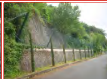
Sistema di barriere paramassi
