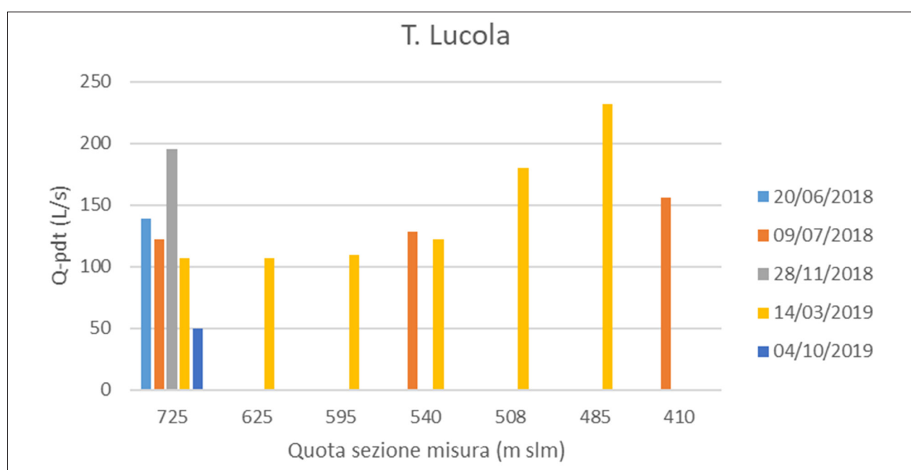
Figura 5 – Misura di portata in diverso tempo e a diverse quote nel T. Lucola.
