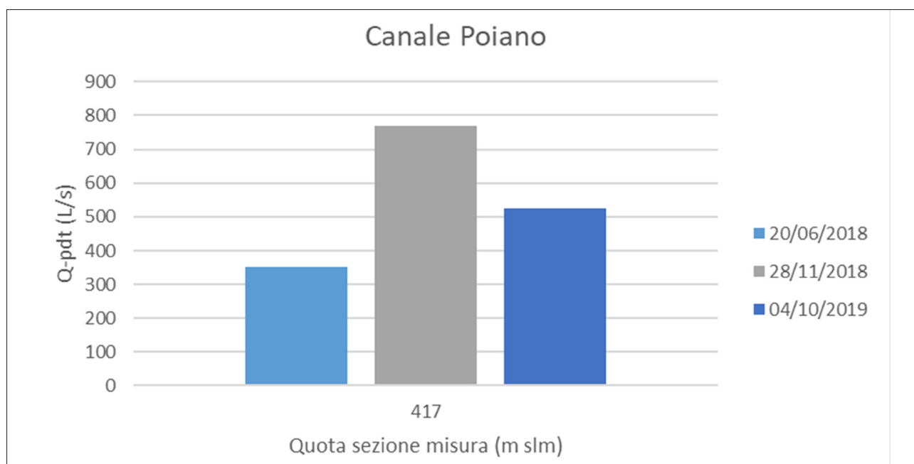
Figura 4 – Misure di portata nelle Fonti di Poiano in date differenti.
