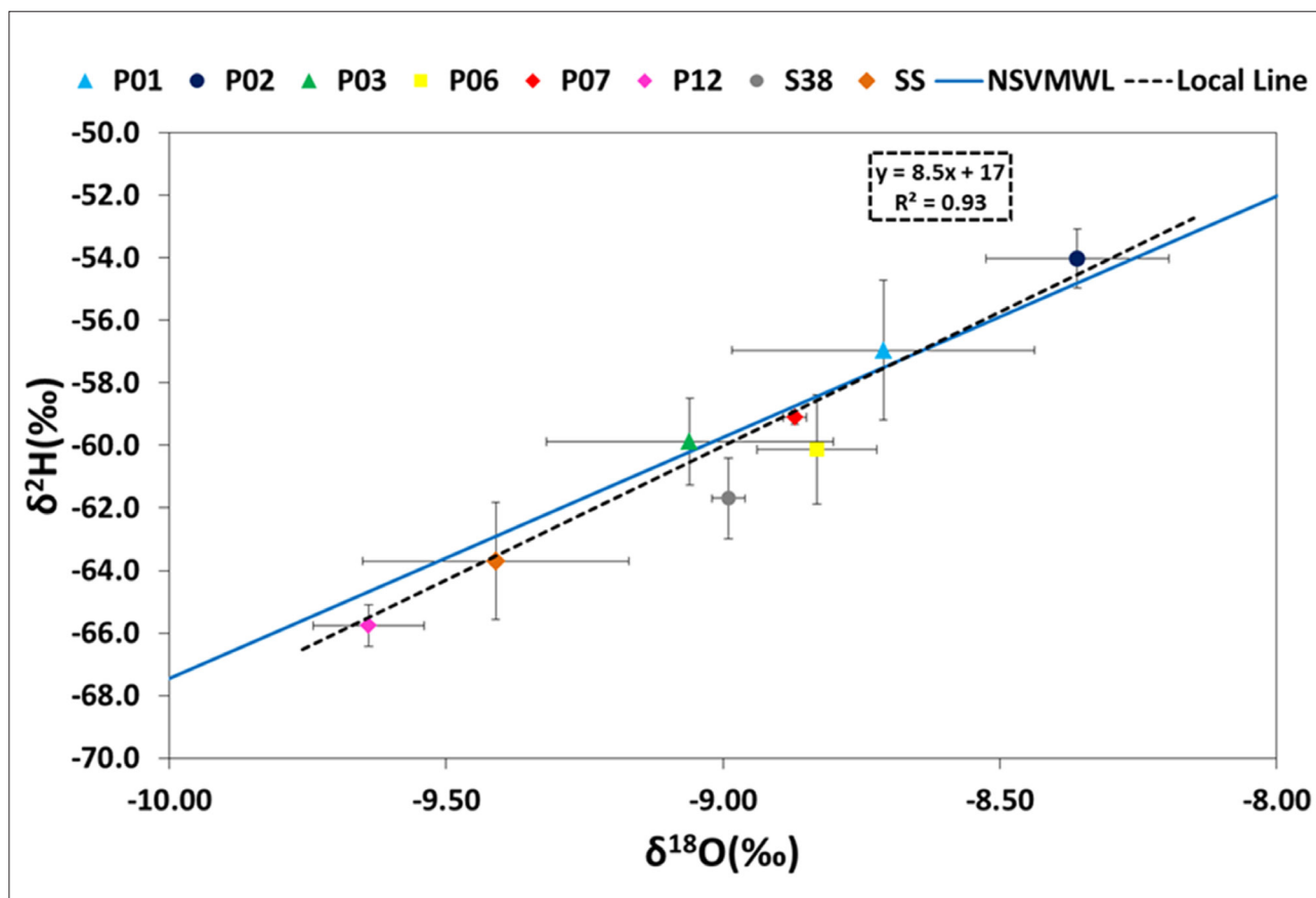
Figura 7 – Grafico \delta^{18}\text{O} - \delta^2\text{H} dei valori isotopici medi calcolati per ciascun punto di campionamento (Figura 1). Per ciascun punto sono riportate le barre di deviazione standard. Legenda punti di campionamento: T. Ozola, I.Oz; F. Secchia, I.Se; F. Secchia dopo confluenza con Ozola, I.Se+Oz; Rio Sologno, I.So; T. Lucola, I.Lu; Fonti di Poiano, I.Po; Sorgenti superficiali, I.Ss; Sorgente Tanone, I.Ta.
