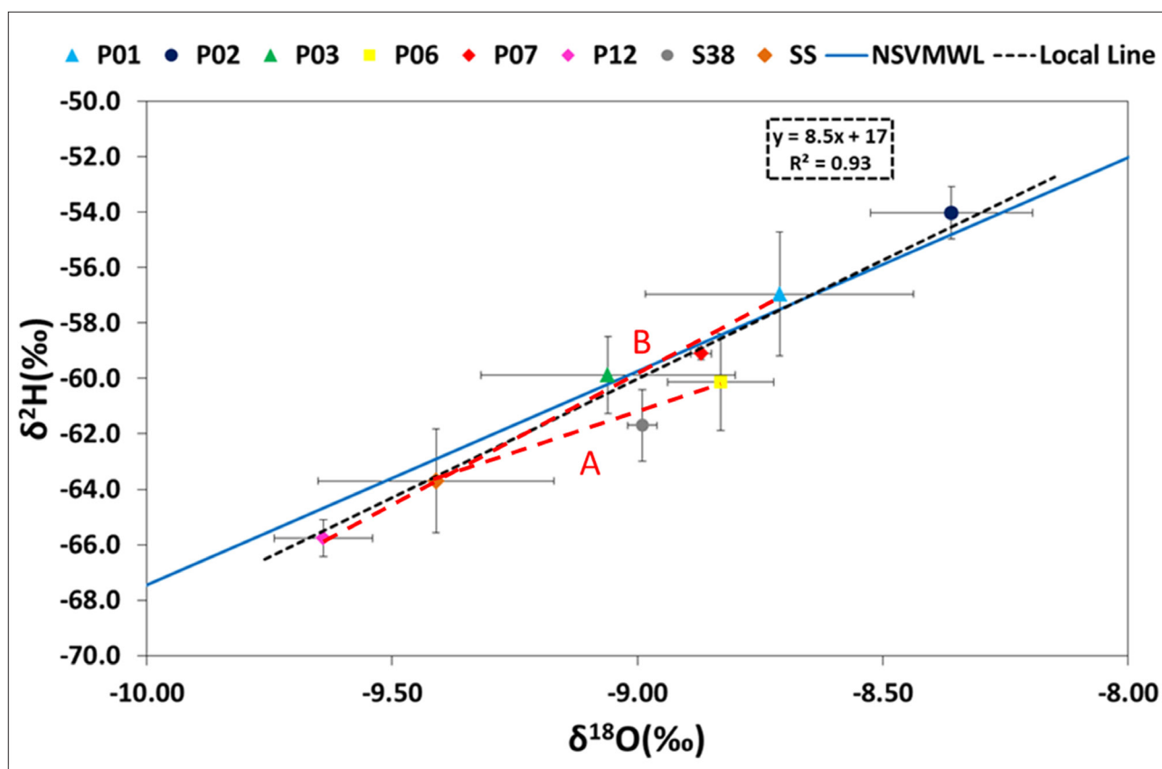
Figura 8 – Grafico \delta^{18}\text{O} - \delta^2\text{H} dei valori isotopici medi calcolati per ciascun punto di campionamento (Figura 1). Nella figura sono state aggiunte le possibili linee di mescolamento per comprendere il bilancio di massa (isotopico) che stabilisce l'alimentazione della risorgente del Tanone (linea rossa A) e l'alimentazione delle Fonti di Poiano (linea rossa B).
